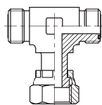
7762 T-Образный ORFS vk – ORFS vk – ORFS sk
