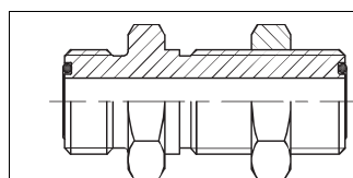
7705 Через переборку ORFS vk – ORFS vk
