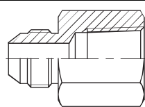
7650 J GAI Внутр. резьба – NPTF sk
