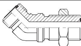
7707 Угловой 45° ORFS vk – ORFS vk
