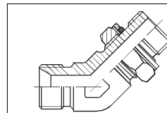
7210 G vk – R vk
