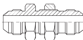
7605 Прямой фитинг для соединения через переборку
