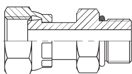
7767 ORFS sk – UNF vk
