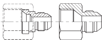
7670 J EVGE Переходник с гайкой
